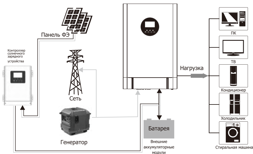
Рис. 1 Энергосистема инвертора
