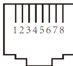
DRM Port
